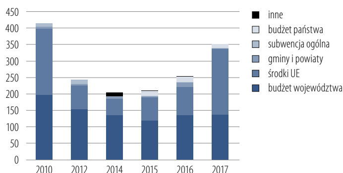
Wykres 148. Nakłady finansowe przeznaczone na drogi wojewódzkie (w mln zł)
