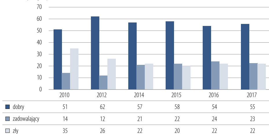
Wykres 147. Stan techniczny dróg wojewódzkich 2017 (w %)
